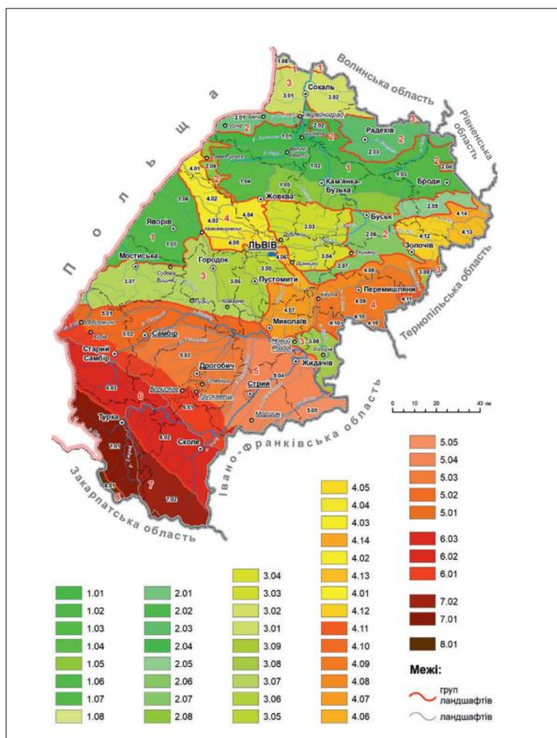
Рис. 2.6. Ландшафтна карта Львівської області
